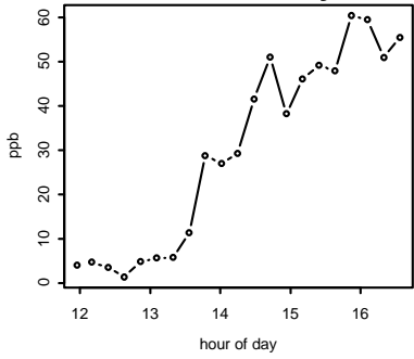
apinene
